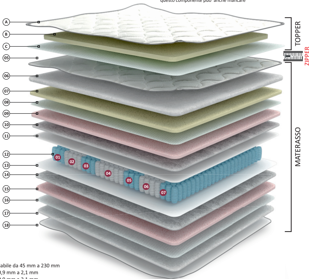
10 - 14 Peso variabile da 300 g/m 2 a 1500 g/m 2 Spessore variabile da 3 mm a 15 mm questo componente puo' anche mancare
